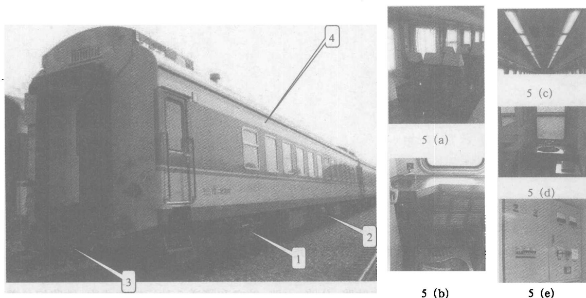
图 1-1 车辆组成
