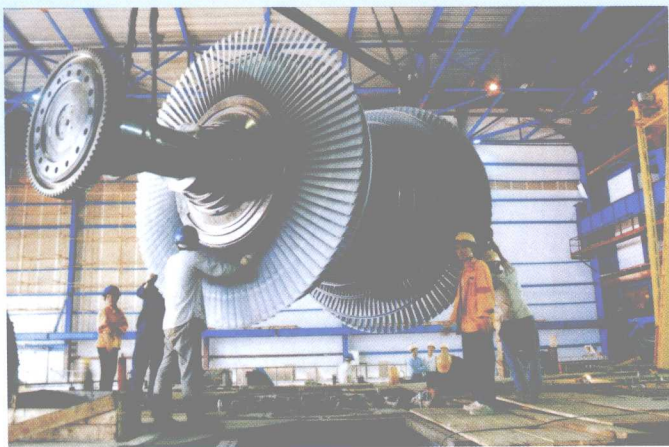
1995年华能汕头电厂1号发电机组（30万千瓦）的汽轮机转子在安装
