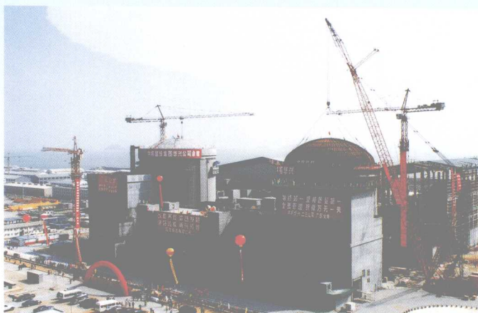
2000年7月,岭澳核电站1号机组穹顶在吊装
