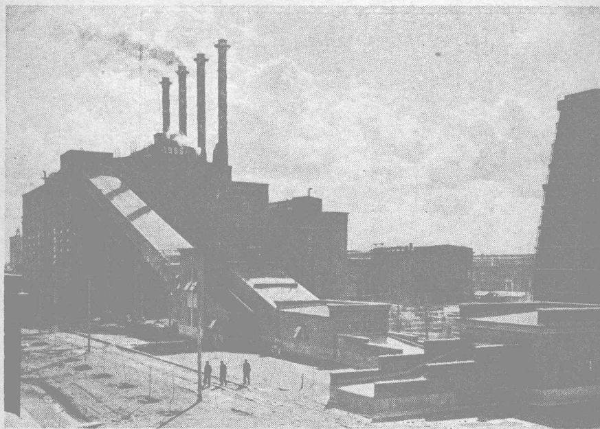
这是第一汽車制造厂动力系統的主要組成部分——热电站的外景。
