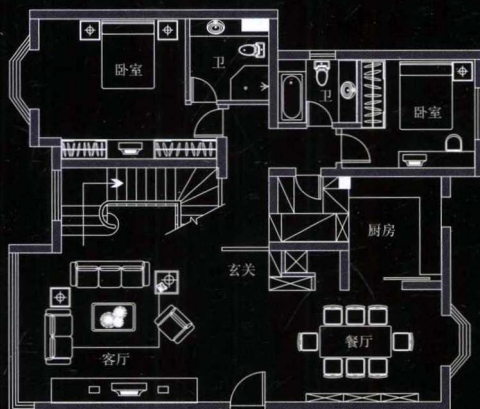
一层平面布置图
