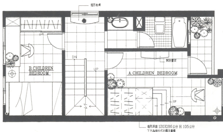
二楼平面配置图
