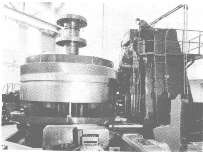
图 1-1 正在加工汽轮机用齿轮的滚齿机
