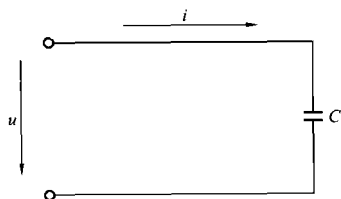
图 1-4 交流电容回路
