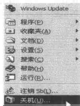
图 2.7 “开始”菜单
