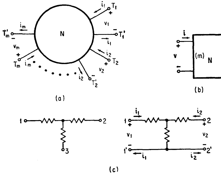
图 2.2.1 用有关端口表示的网络
