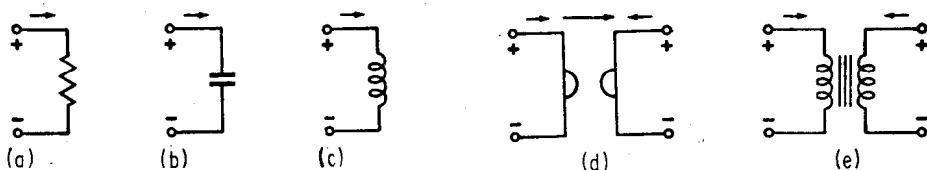
图 2.2.2 基本电路元件的表示法及其定义
