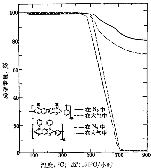
图1 聚苯并咪唑的热失重曲线
