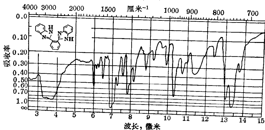
图2 聚苯并咪唑及模
