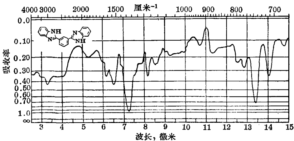
拟化合物的紅外光譜
