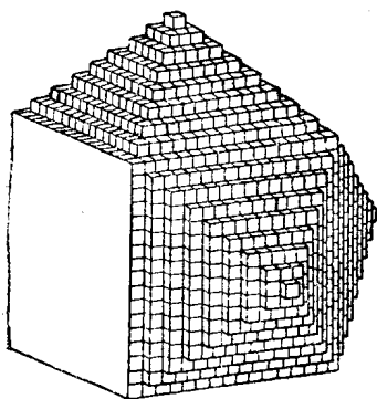
圖 4. 由於構造單位(立方體)的數目的減少而產生了新的晶面。
