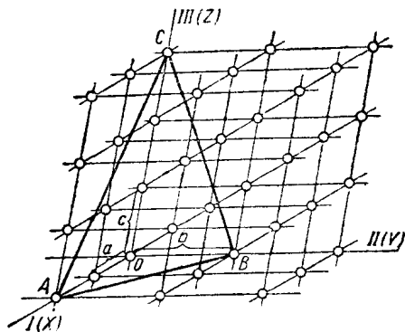
圖 2. ABC 晶面在坐標軸上截整數間距。
