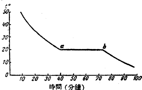
圖 7. 結晶物質的冷卻曲線。
