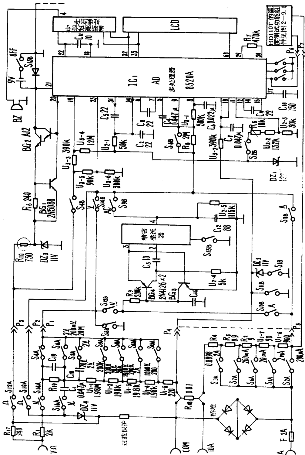
HD100/HD110 型数字万用表
