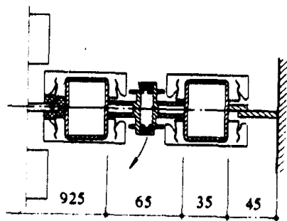
C - C
