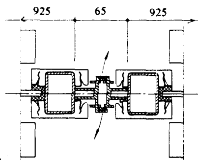
B - B
