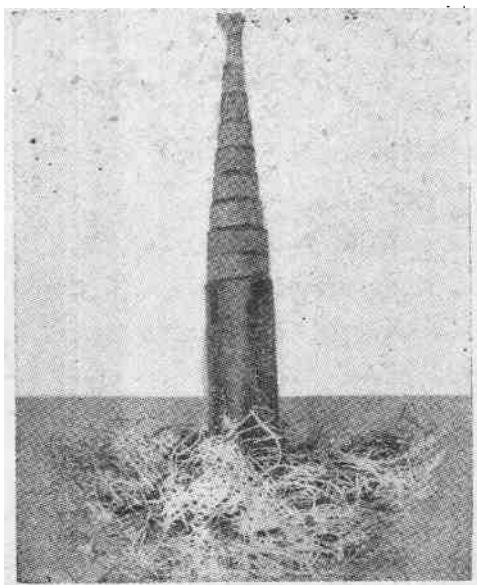
圖 2 城市愈發達，電線愈來愈多，空中架不下，於是另用新式的電纜。這是 2400 根電線扭成的電纜，直徑不過 7.5 公分，埋在地下，比將 2400 根電線架在空中方便得多了。
