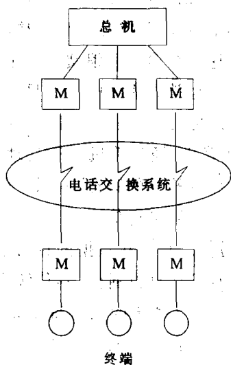
图 1-1 联机通信系统
