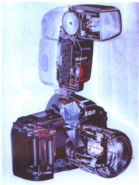
图 5 先进的尼康 F90 照相机
