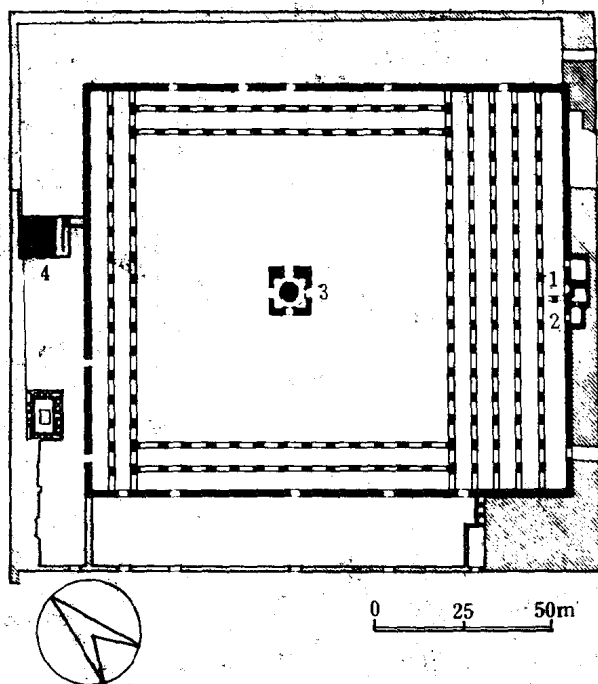
图3 埃及开罗伊文士伦清真寺平面图
