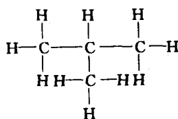
异丁烷(具有支链)
