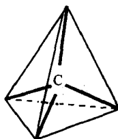
图 1-1 碳原子价键正四面体结构
