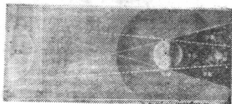
图四 日蚀成因图
