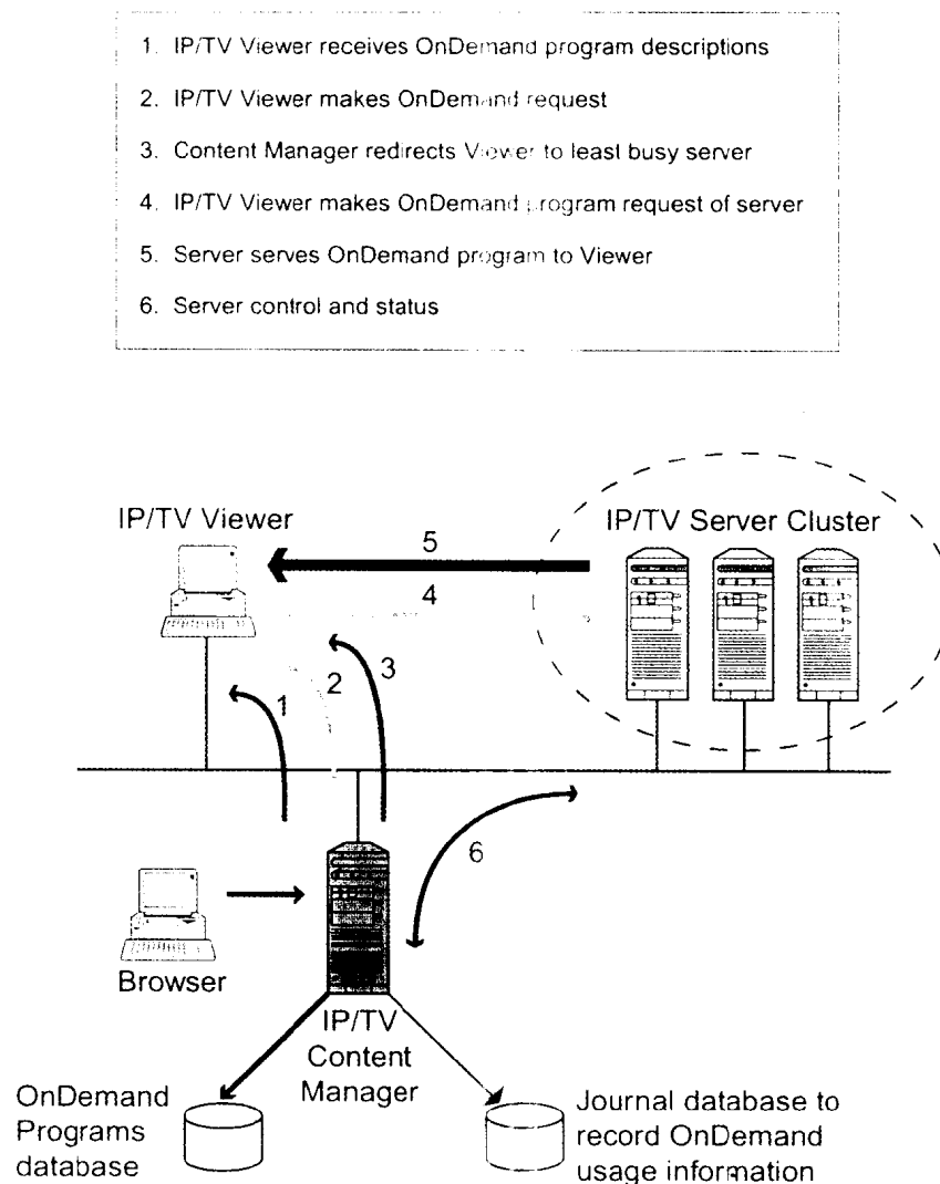
图 1-2 IP/TV 部件——点播节目
