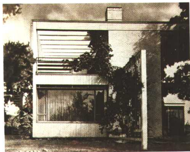
附图12 格罗皮乌斯: 格罗皮乌斯自宅西立面(1936)
