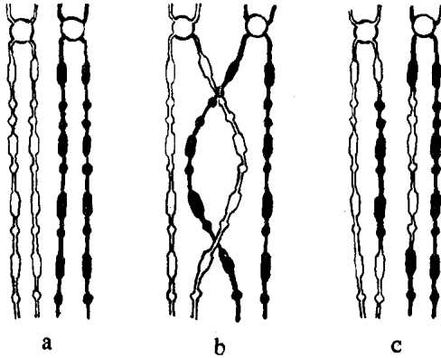
图 1.4 在成熟的生殖细胞发展的一个时期里,一对染色体(见 a)的两个成员互相接近而且变成紧密交织(见 b)。在这个时期里,一个染色体的一节也许与另一个染色体的相当一节交换了,因此,当这一对重新分开时(见 c),我们得到了两个染色体(比较 a 及 c)的基因的新组合。这种现象叫做“基因交换”。
