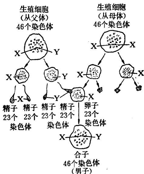
图 1.3 成熟的双亲生殖细胞与合子的关系。父亲与母亲两者每个成熟的生殖细胞(图解的顶端)有染色体的全数(23对,或 46 个染色体)。当这些生殖细胞达到完全成熟,它们经过分裂而变成卵(对女的而言)与精子(对男的而言)。在典型情况下,卵中只有一个是充分发展了的且能受精,其它的是不起作用的。
