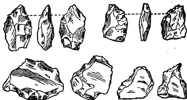
在基克一科巴洞（克里木）底层发现的 苏联旧石器时代最古的一些石器
