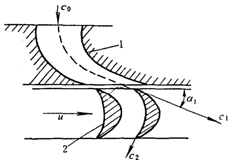
图 1-1 冲动级汽道中蒸汽流动情况
