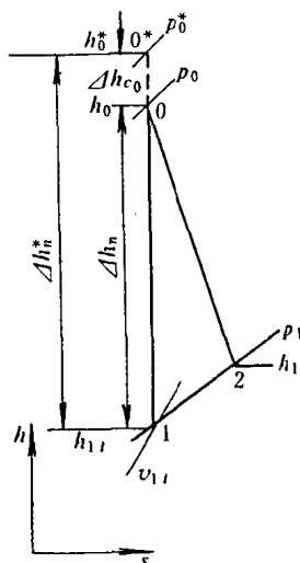
图 1-7 蒸汽在喷嘴中的热力过程
