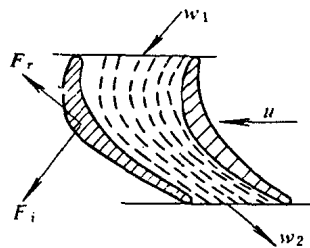
图 1-2 蒸汽在动叶汽道内
