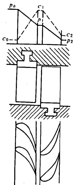
图 1-5 反动级中蒸汽压力和速度变化示意图
