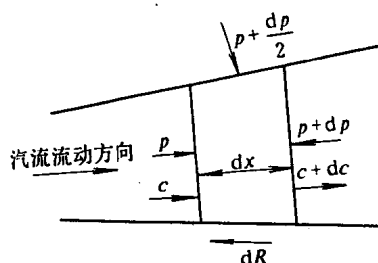
图1-6 作用在汽流微段上的力
