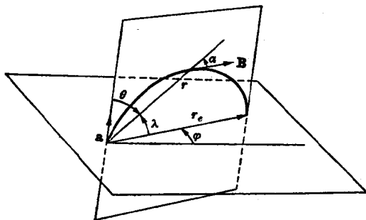
图 1.1 偶极子 \mathbf{a} 的磁力线
