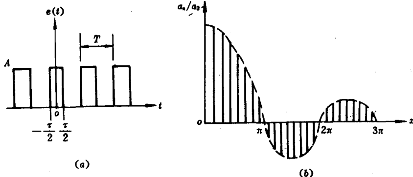
图 2.5 周期性脉冲及其频谱
