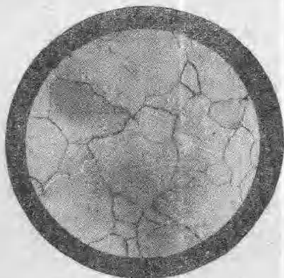
圖 1 純銅的顯微結構( \times 200 )
