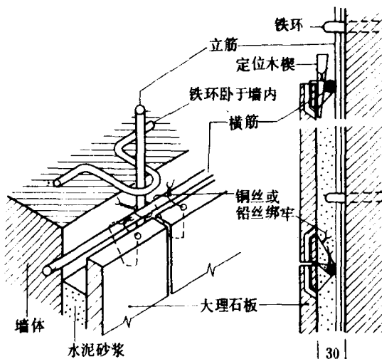
图 1-1 大理石安装法
