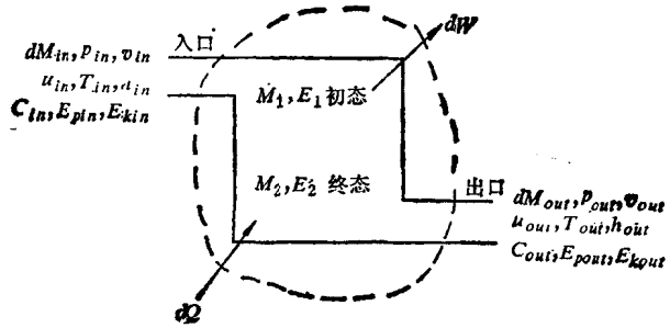
图1-1 非稳态、非稳定流热力系统图
