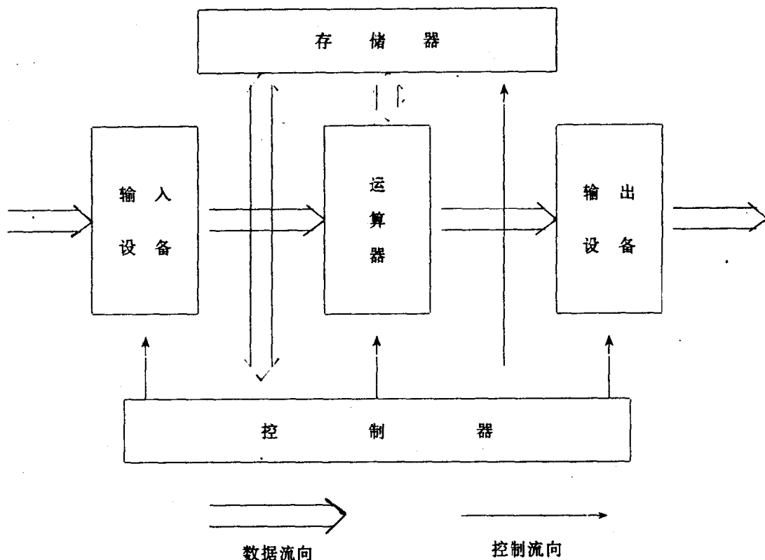
图1.2 计算机硬件结构框图
