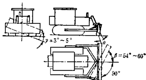
图 1-5 推土机推土刀角度的调整
