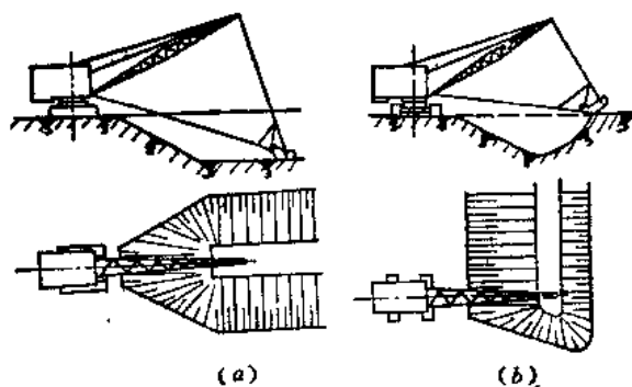
图 1-2 拉铲挖掘机的开挖方式 (a)正向开挖; (b)侧向开挖
