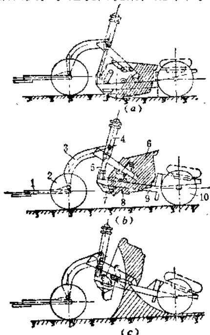
图 1-3 牵引式液压操纵铲运机的工作过程
