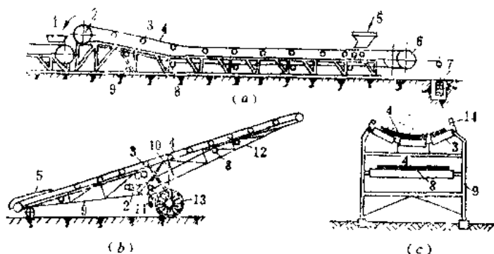
图 1-8 带式输送机
