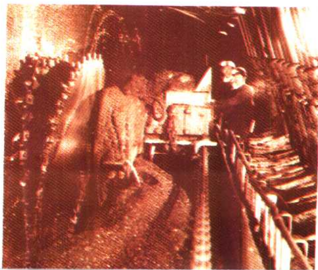
七星煤 矿综合采煤 机组工作面
