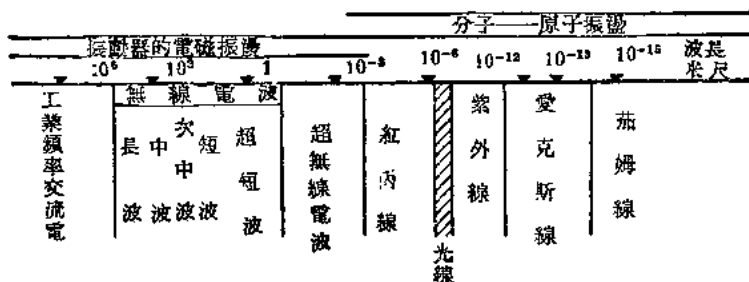
圖 1-1 輻射譜
