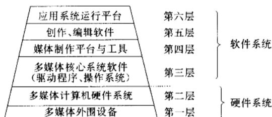
图1.2.1 多媒体系统的层次结构
