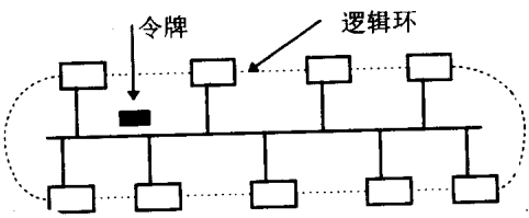
图 1.9 令牌总线的工作原理
