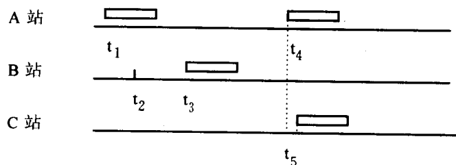
图 1.7 CSMA/CD 的工作原理
