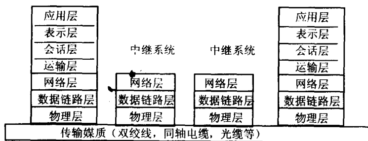
图 1.5 计算机网络的体系结构——ISO/OSI 参考模式
