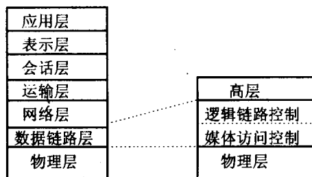
图 1.6 局域网体系结构与 OSI 体系结构的对照
