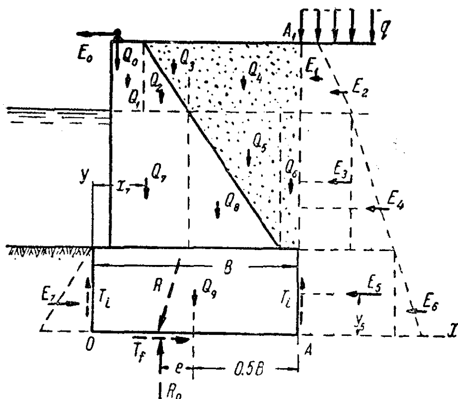
圖 5. 擋土牆上及其基礎上的力的作用圖
