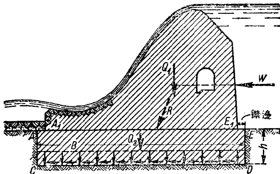
圖 2. 滾水壩的橫断面 ACDE—基礎； AA_1 和 EE_1 —襟边
