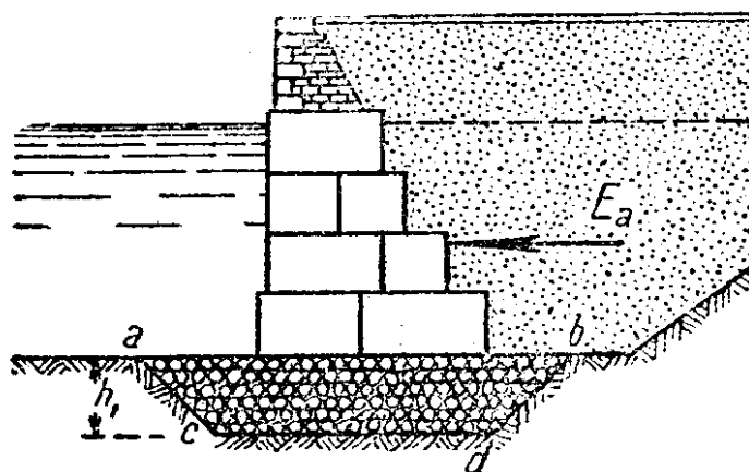
圖 4. 駁岸牆土牆的橫断面 acdb—圓石人工地基
