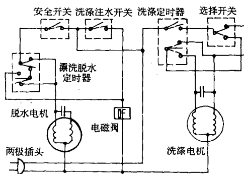
双马牌 XPB20-S 型洗衣机
