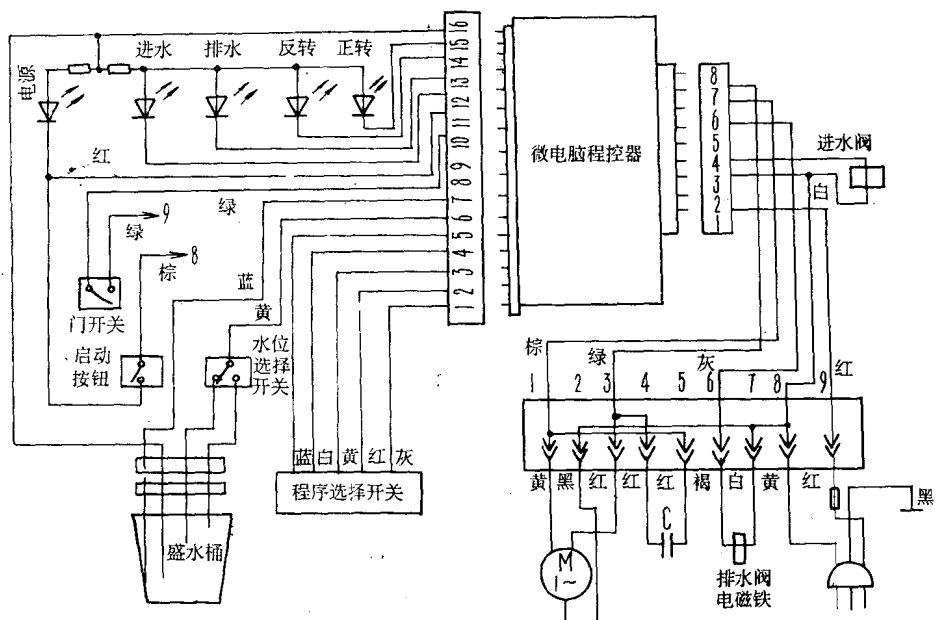
申花牌 XQB30-1T 型洗衣机
