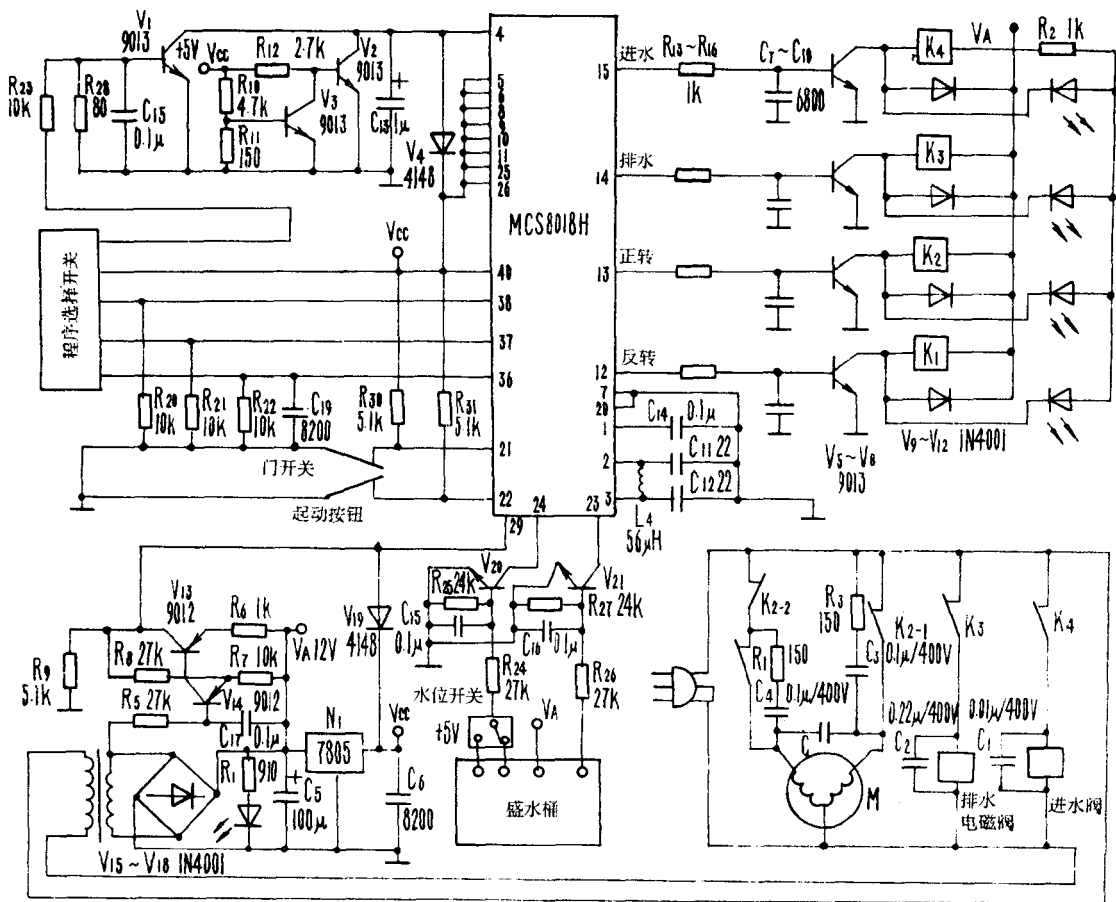
友谊牌 XQB36-1 型洗衣机
