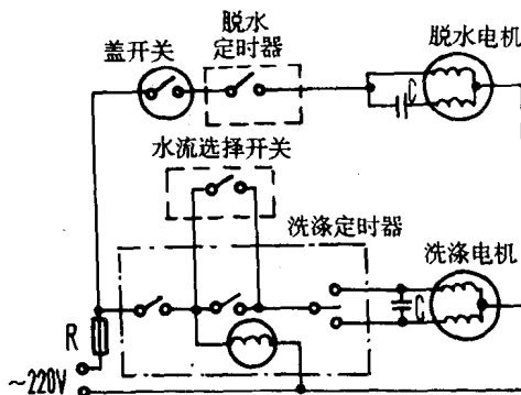
松陵牌 XPB20-2S 型洗衣机
