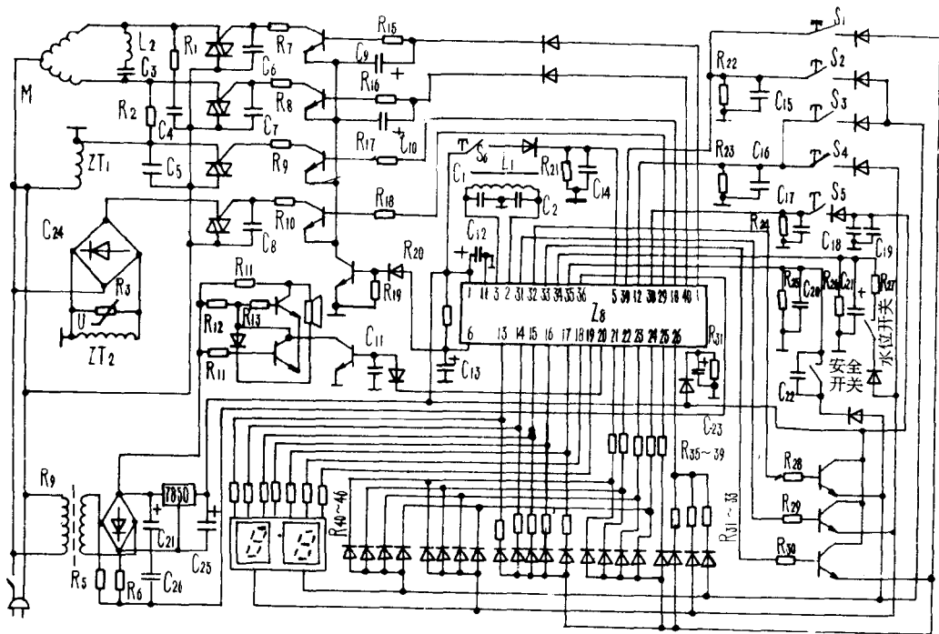
友谊牌 XQB36-1 型洗衣机
