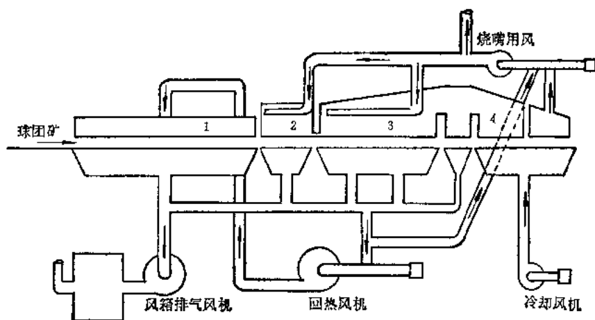
图 1-6 环式球团焙烧机
