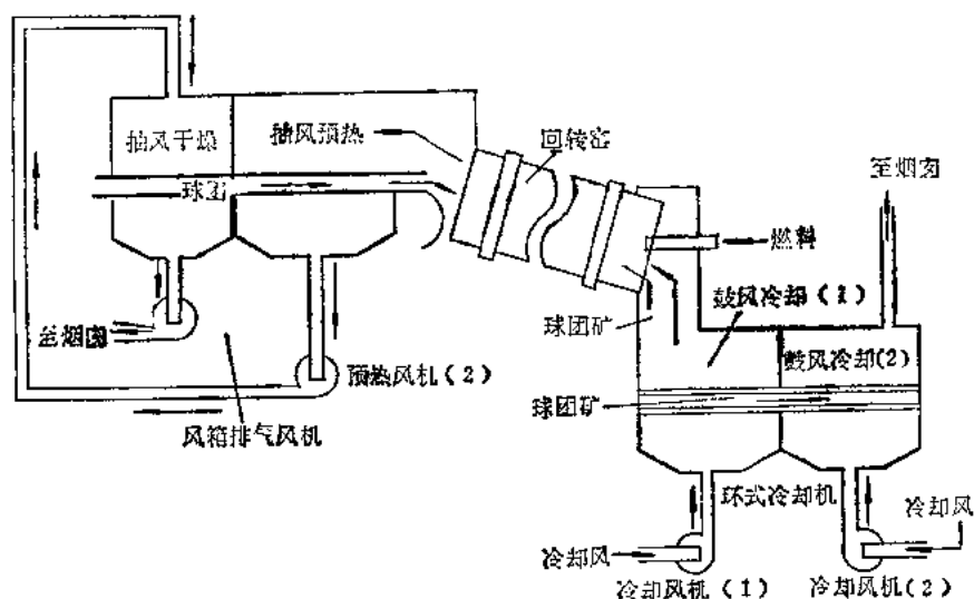
图 1-5 阿里斯-查尔默斯链篦机-回转窑系统采用二次，二区段抽风循环处理赤铁矿
