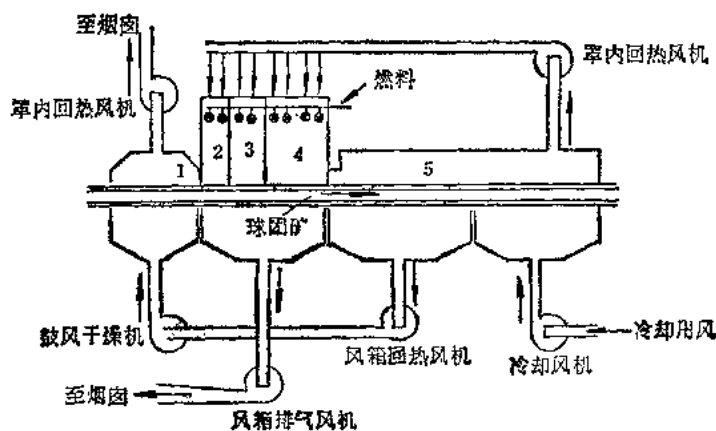
图 1-2 麦基带式焙烧机系统处理磁铁精矿
