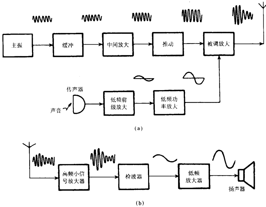
图 0-3 简单的无线电广播发送和接收系统方框图
