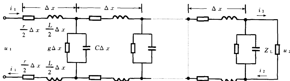
图 1-1 均匀传输线
