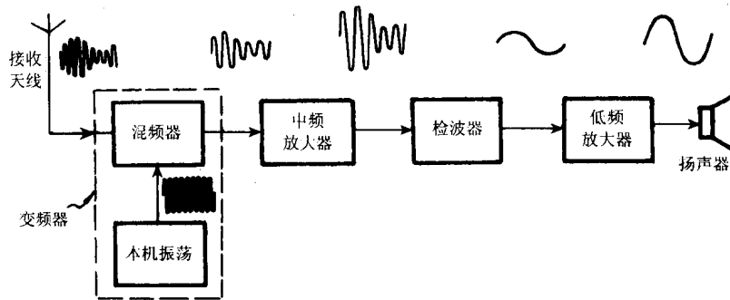
图 0-4 超外差式接收机方框图
