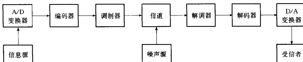
图 0-5 数字通信系统组成方框图
