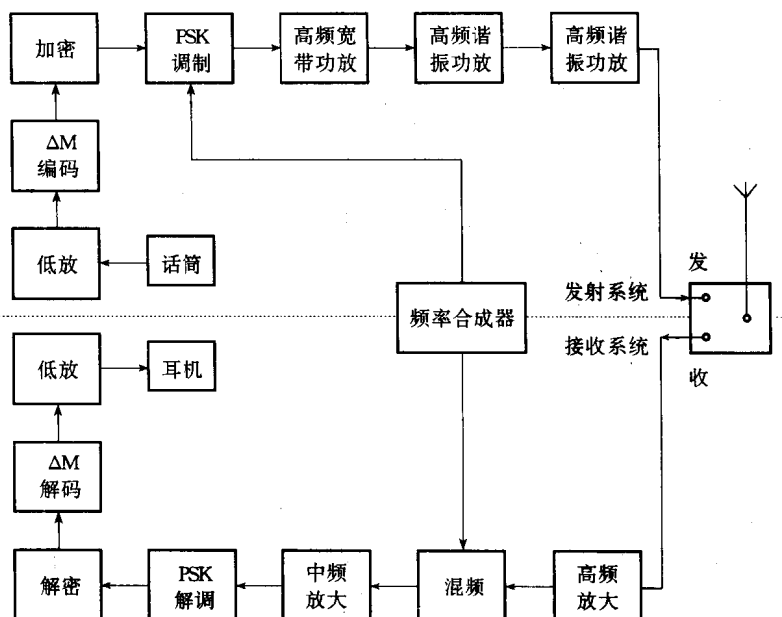
图 0-6 典型数字通信机组组成方框图
