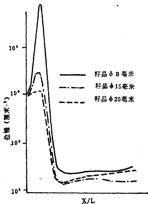
图2 三温区法接籽晶生长的 GaAs 单晶位错密度分布情况( \phi 30 毫米)
