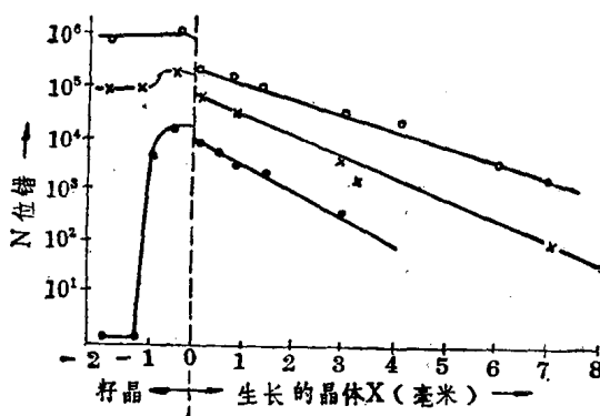
图3 直拉法结晶中的位错与距离的关系
