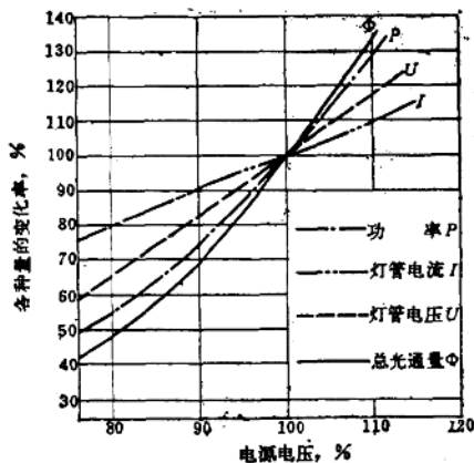
图 39-2-8 电源电压变化对 400 W 高压钠灯光电参数的影响
