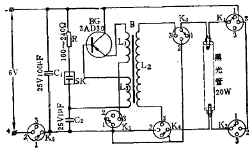
图 39-2-13 单管式电源变换器线路
