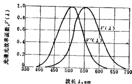
图 39-1-2 光谱光效率函数
