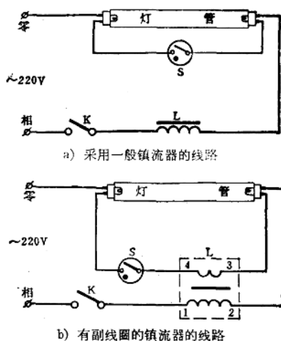
图 39-2-3 预热式荧光灯工作线路
