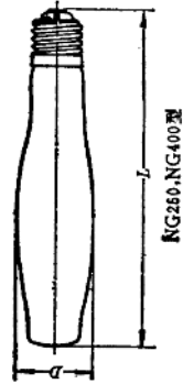
外 形 图
