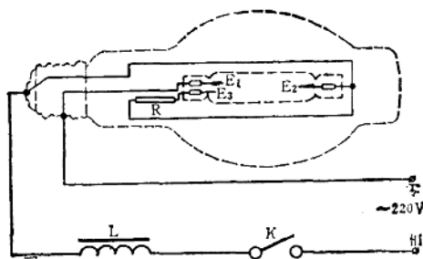
图 39-2-5 荧光高压汞灯工作线路
