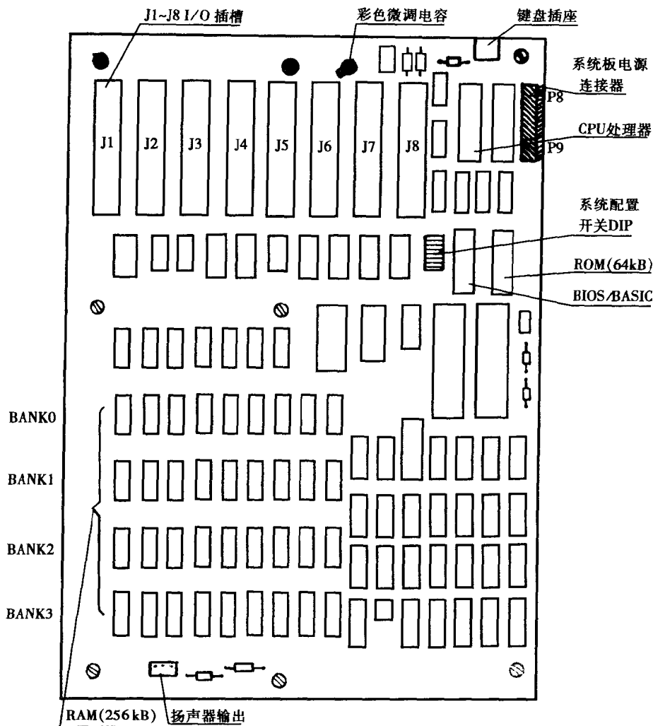
图 1.3 系统板元件布置图
