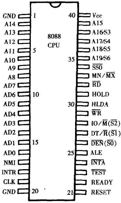
图 1.4 8088 CPU 引脚排列
