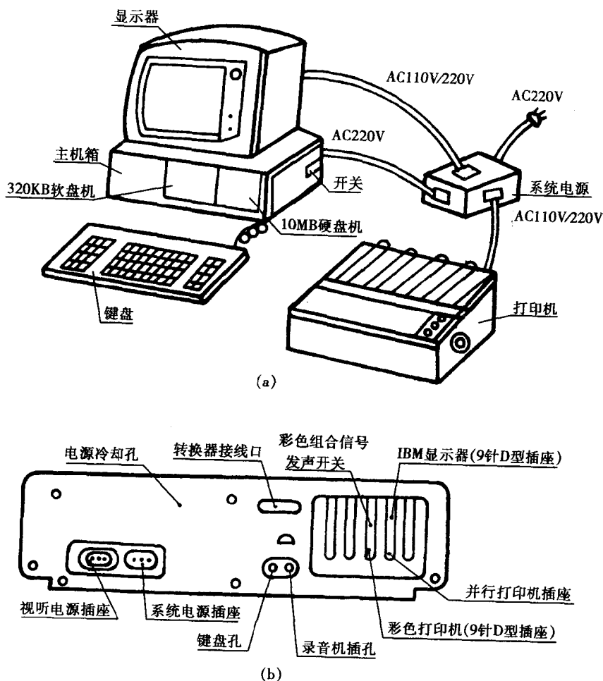
图 1.1 IBM PC/XT 微机系统装配示意图 (a)系统各部件装配示意图 (b)系统背面接线图
