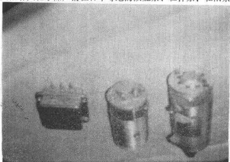
贵阳小河电工厂生产的各种摩托车电动机
