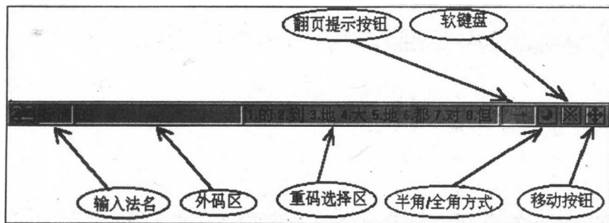
图 1-4 中文输入法提示行
