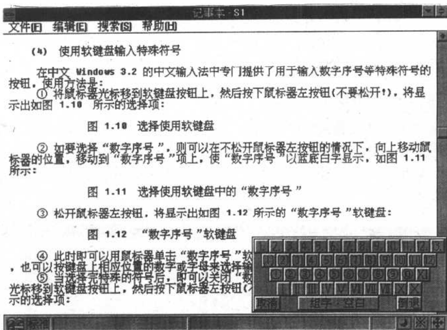
图 1-10 “数字序号”软键盘
