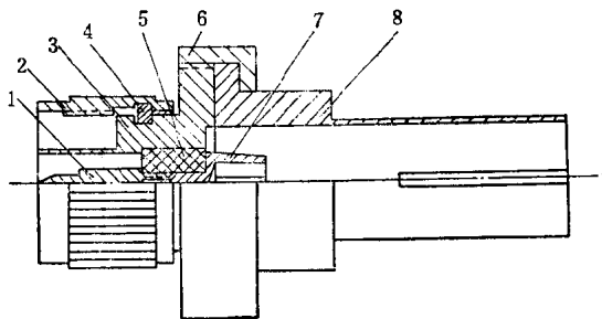
L16 型接头
