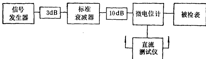
图3 1mV以下电压校准连接图
