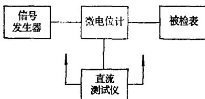
图2 1~100 mV 电压校准连接图
