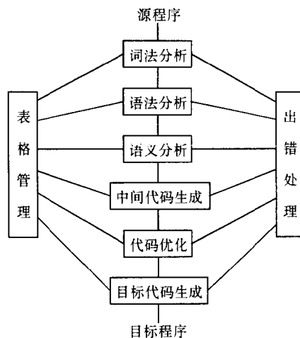
图 1.3 编译的各个阶段
