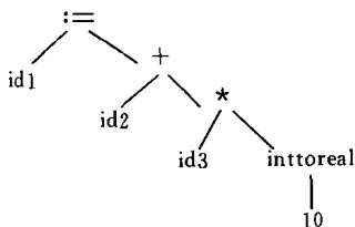
图 1.6 插入语义处理结点的树
