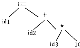
图 1.5 语句 id1 := id2 + id3 * 10 的语法树的另一种形式
