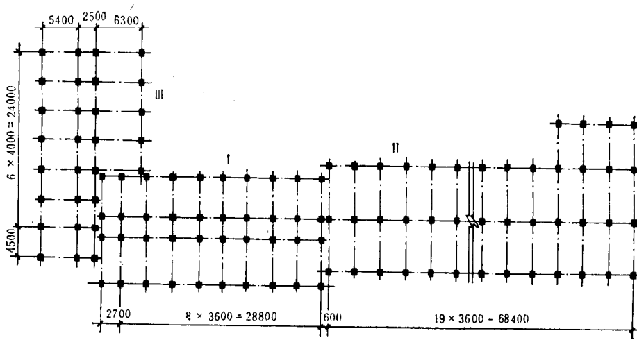
图1-4 北京民航大楼框架柱网布置
