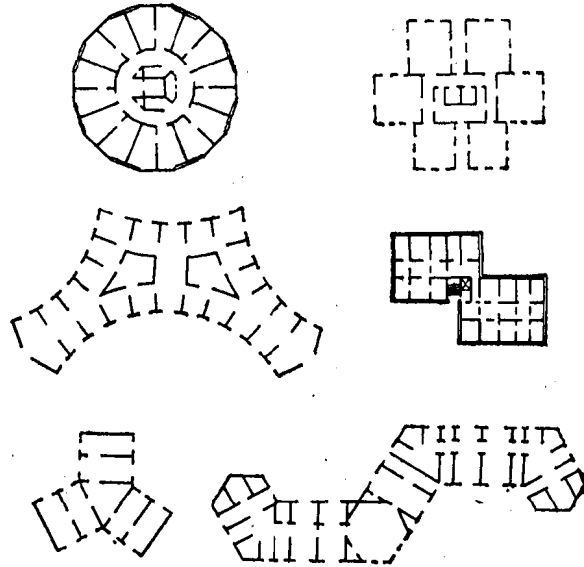
图1-6 剪力墙结构平面布置举例
