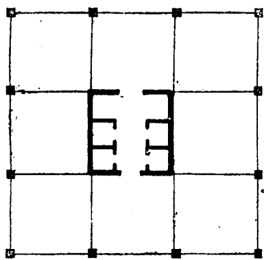
图1-11 框架-筒体结构的典型布置
