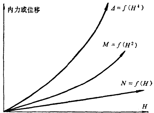
图1-1 结构内力、位移与高度的关系
