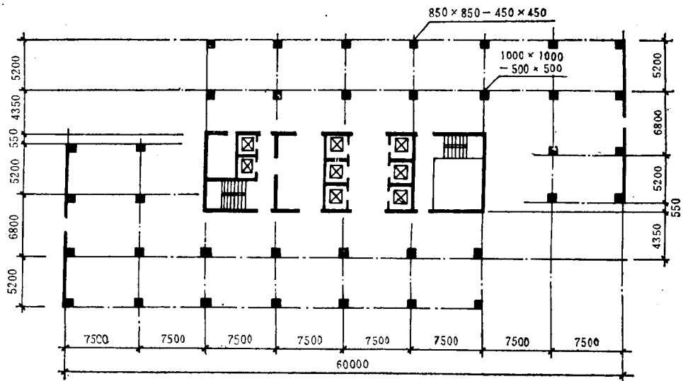
图1-10 上海宾馆平面布置
