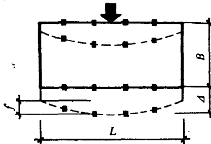
图 1-13 楼板水平变形
