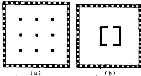
图 1-14 框筒及筒中筒结构典型平面
