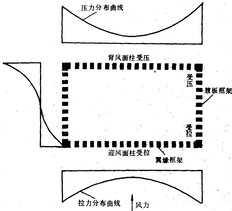
图1-15 水平作用下框筒柱轴向力分布
