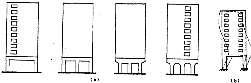
图1-7 框支剪力墙
