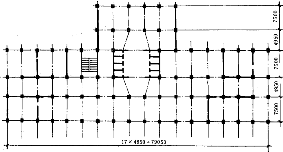
图1-9 北京饭店平面布置
