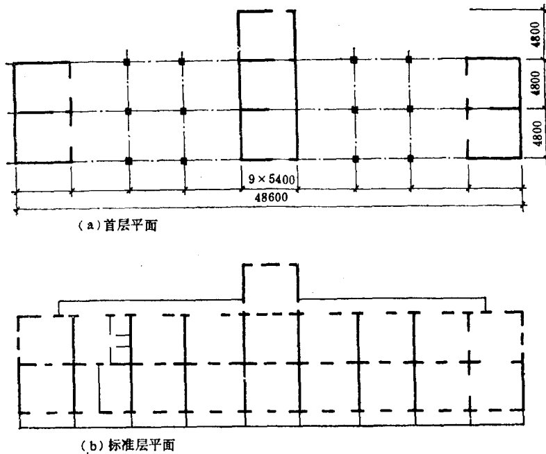
图1-8 底层大空间剪力墙结构
