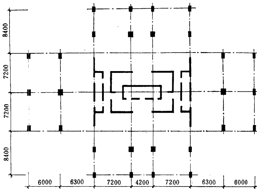
图1-12 上海雁荡大厦结构平面
