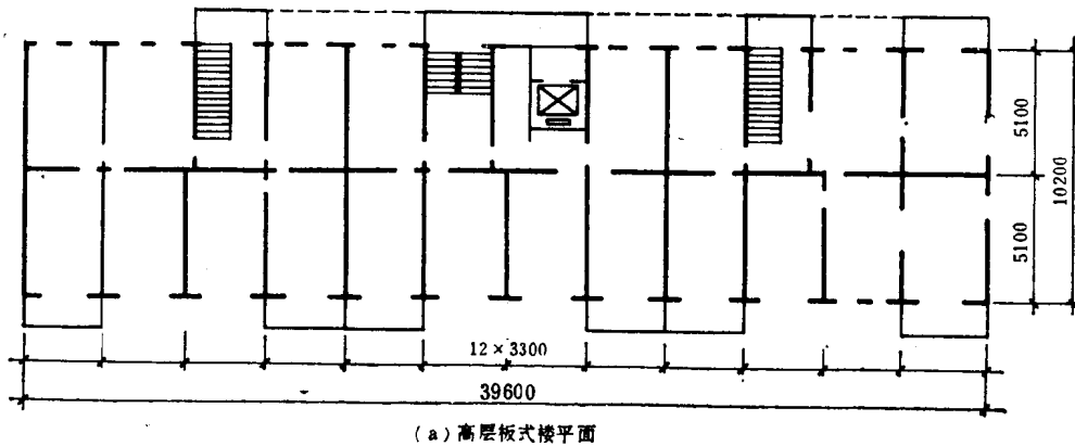
图1-5 剪力墙结构的平面
