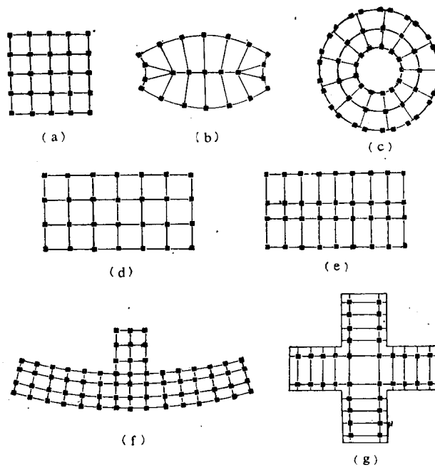
图1-3 框架柱网布置举例
