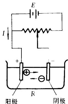
图 1.2 电解池回路
