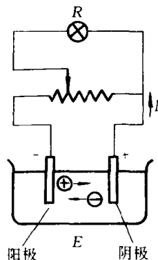
图 1.3 原电池回路
