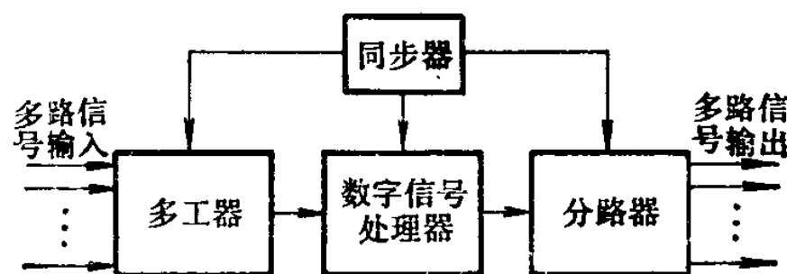
图2 多路信号数字处理系统
