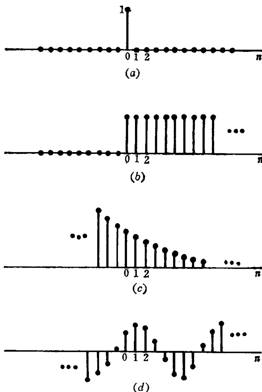
图1.3 a 几种典型的序列 (a) 单位采样 \delta(n) ; (b) 单位阶跃 u(n) ; (c) 实指数 a^n ; (d) 正弦序列 A \cos(\omega_0 n + \phi) 。
