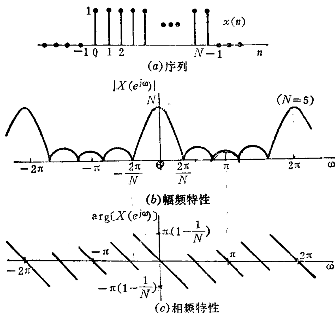
图1.4 等幅有限长序列的傅里叶变换
