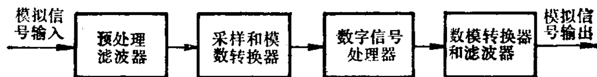
图1 数字信号处理系统基本组成
