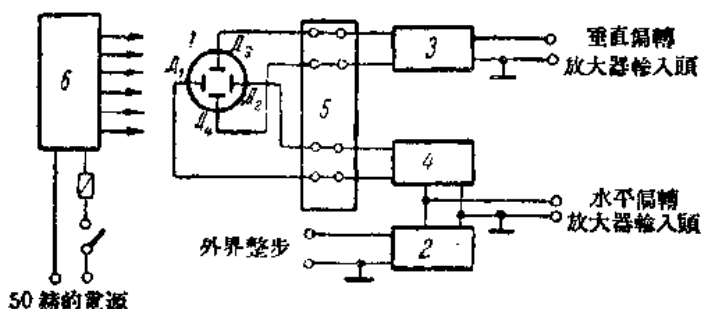
圖1. 陰極射線示波器的方框圖：
