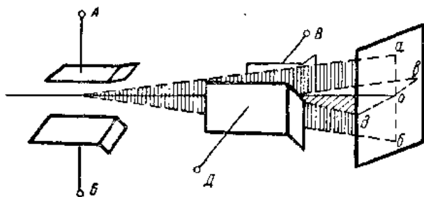
圖6. 陰極射線管的偏轉板極
