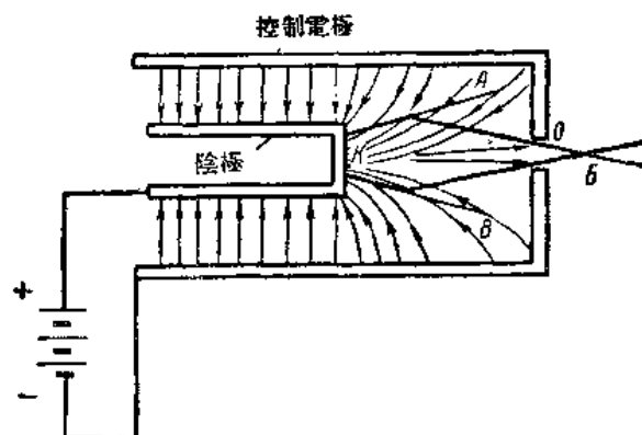
圖4. 控制電極的作用
