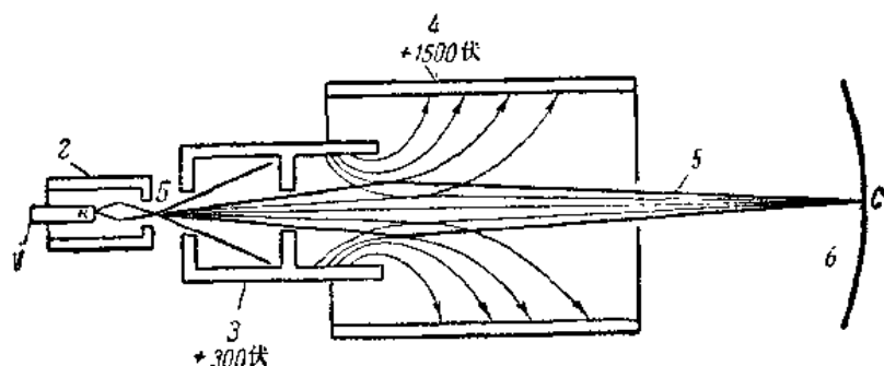
圖5. 在陰極射線管中電子注聚成焦點：
