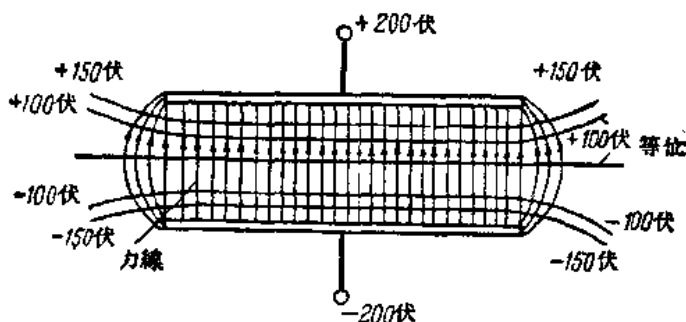
圖3. 兩個平行板極間的靜電場
